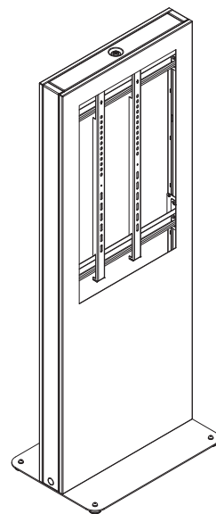
WIDOK IZOMETRYCZNY
