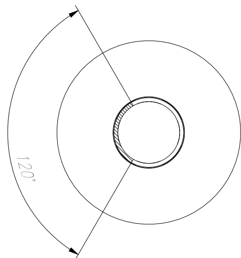
A-A (1 : 2)
